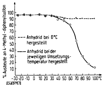
Abb. 1. Sulfonylierung von Benzol mit p -Toluolsulfonsäure-trifluormethansulfonsäureanhydrid (3d) zu 4-Methyldiphenylsulfon (7d) in Abhängigkeit von der Temperatur.
